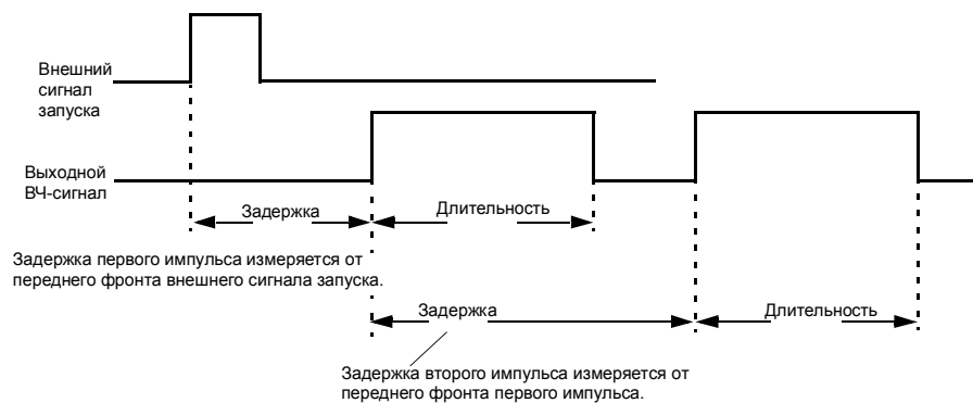
Рисунок 6–2 Настраиваемый дуплет
