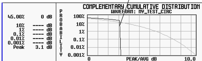
Образец графика сигнала после прямоугольной обрезки
