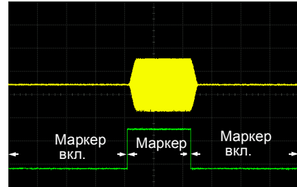
Диапазон выборки начинается в первой точке сигнала
