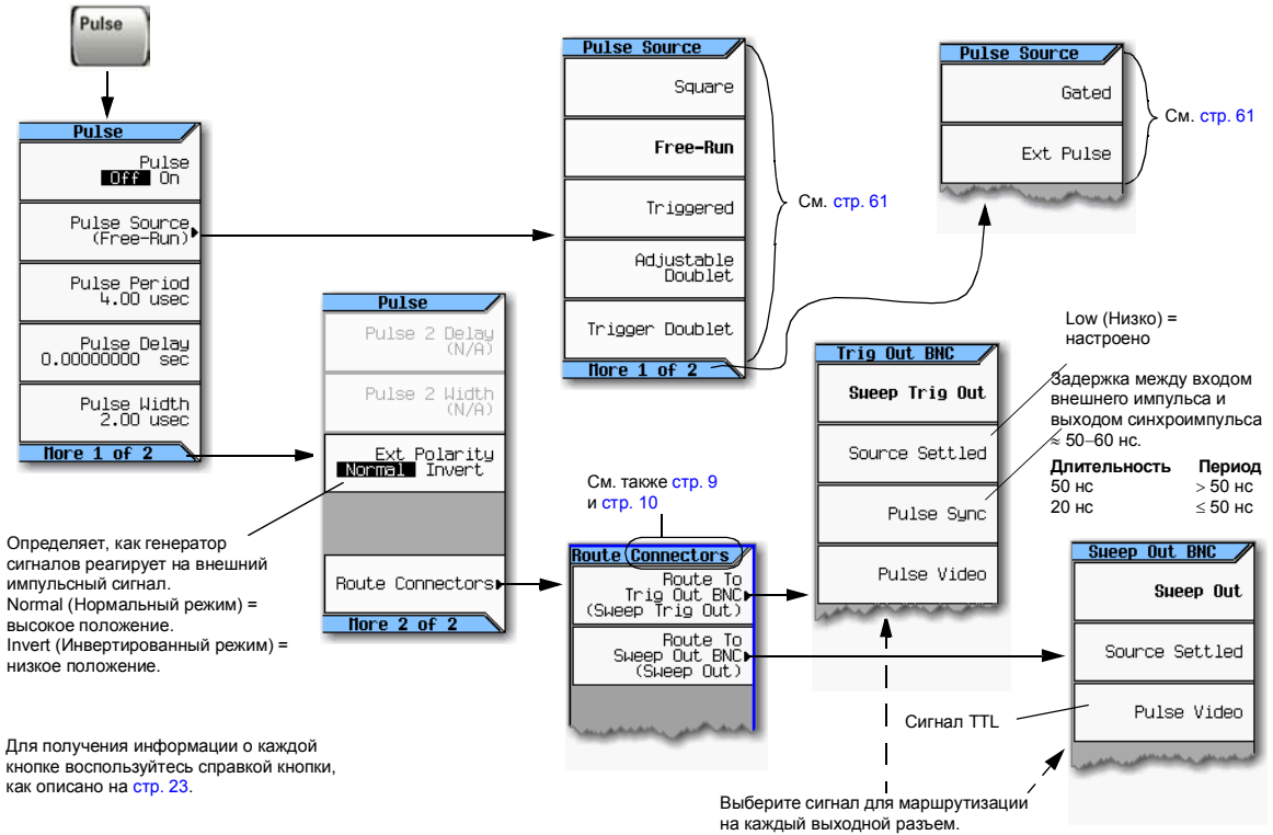
Рис. 6—1 Программные кнопки импульсной модуляции
